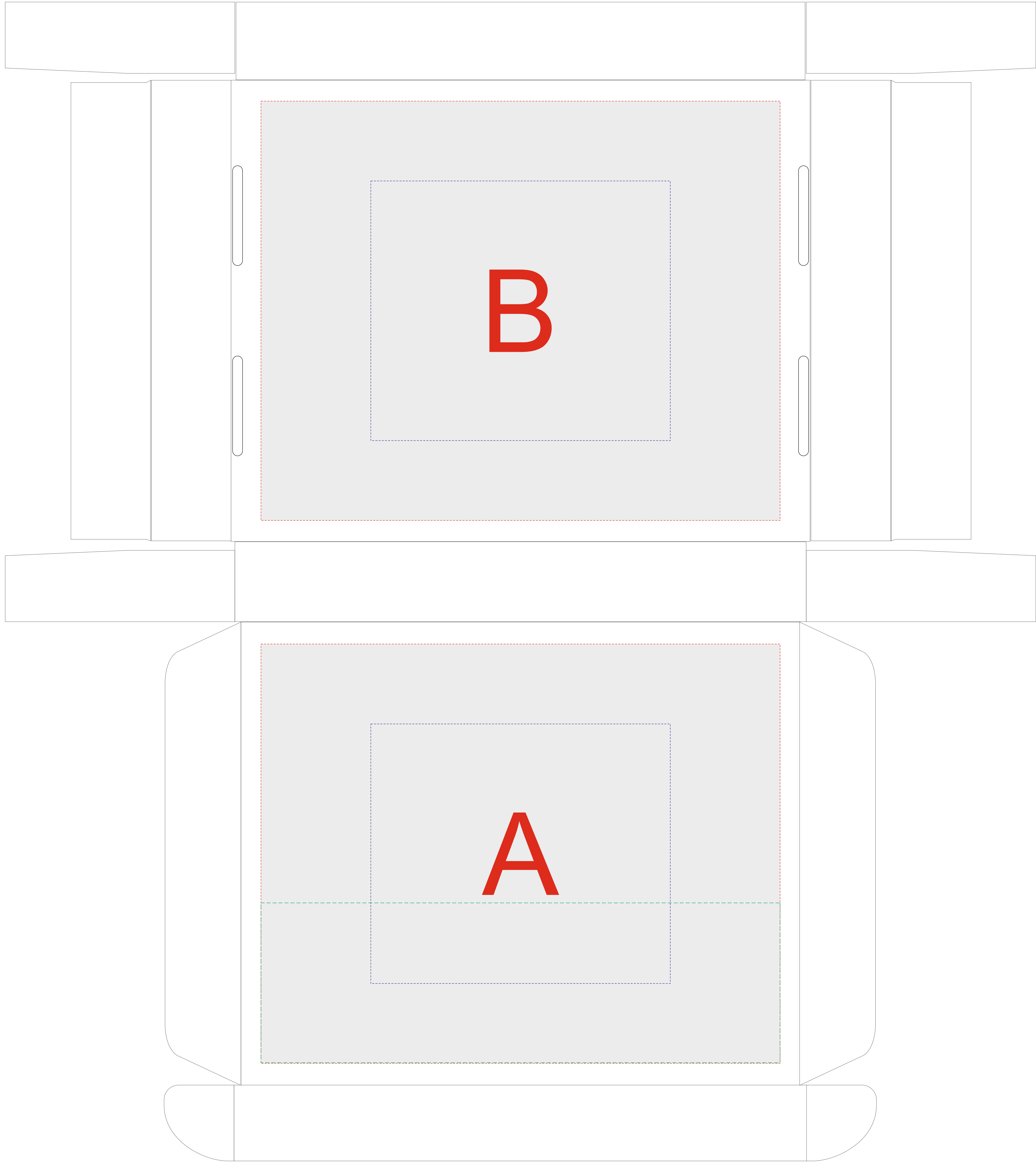
Коробка в разложенном виде ВНЕШНЯЯ СТОРОНА
