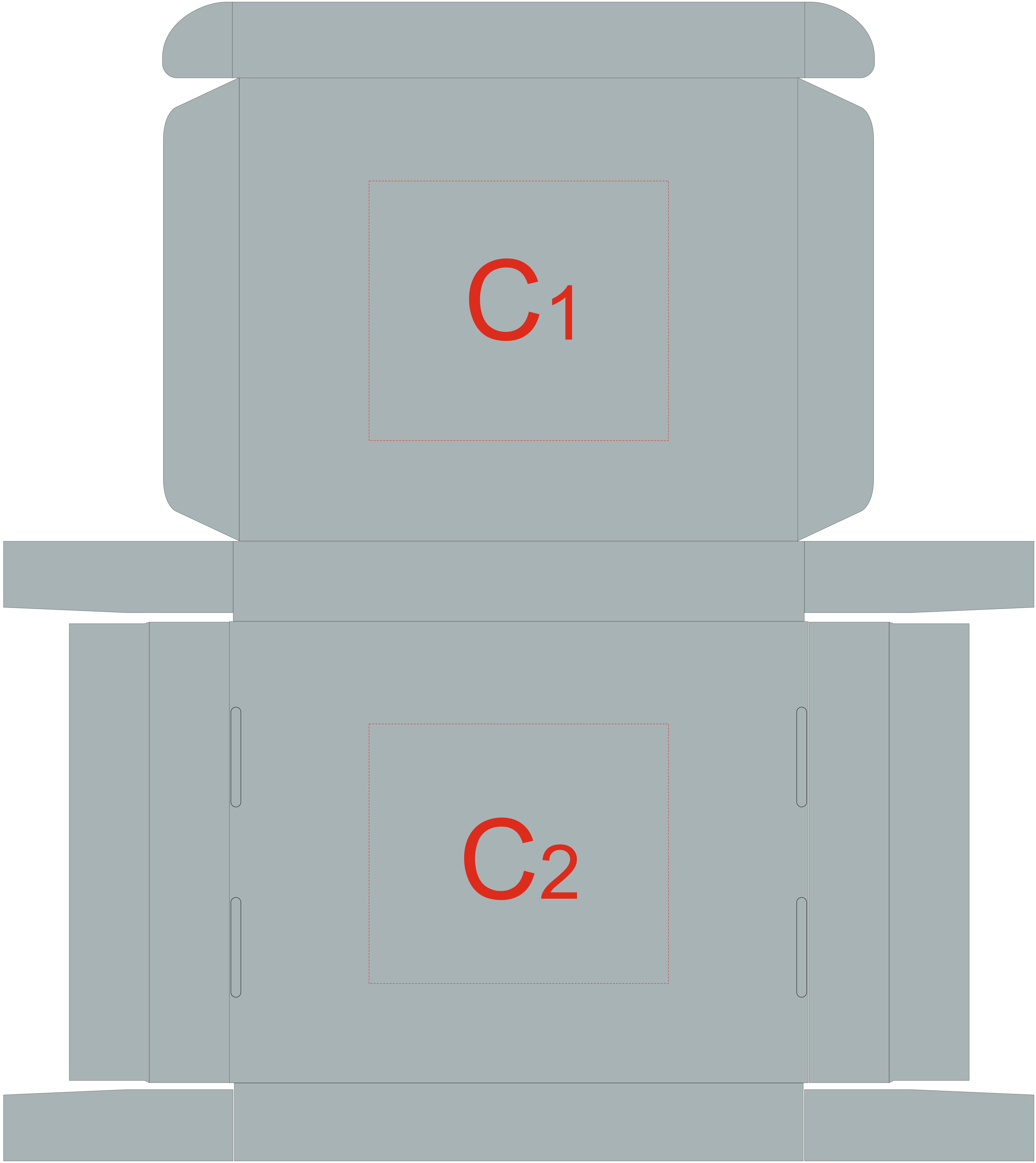
Коробка в разложенном виде ВНУТРЕННЯЯ СТОРОНА
